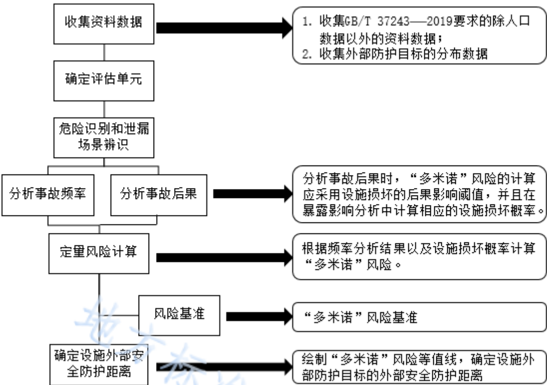
图1 “多米诺”防护设施目标的外部安全防护距离确定方法
