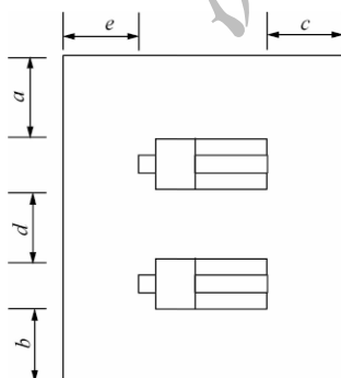
图 6.1.4 机组布置
