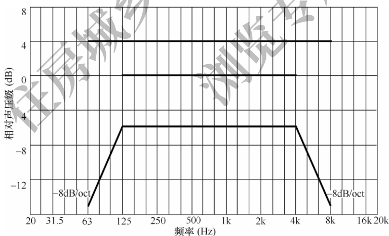
图 20.8.18-2 二级会议扩声系统传输频率特性
