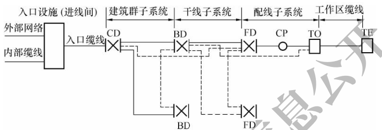
图 21.2.1 综合布线系统构成
